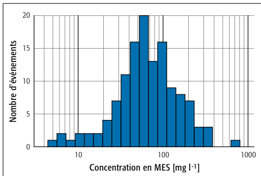
Fig. 2 Distribution des concentrations moyennes en MES par événement de pluie dans les eaux de ruissellement pour 127 événements de pluie dans 7 bassins versants strictement séparatifs en Suisse [8, 9, 10]. La valeur moyenne de cette distribution est de 68 mg/l (cf tab. 1).
