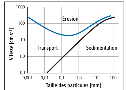
Fig. 4 Critère d'érosion, de transport ou de sédimentation pour des particules uniformes non cohésives [25].
