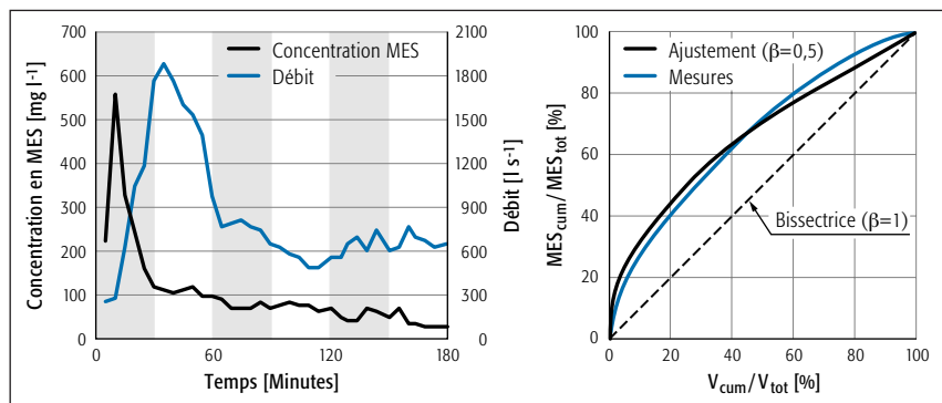
Fig. 3 Evolution des concentrations en MES au cours d'un événement de pluie et évolution de la masse cumulée en MES en fonction du volume d'eau cumulé pour ce même événement (pollutogramme) [16].
